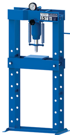
PRENSA HIDRÁULICA 15 TON - BOVENAU
